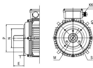
B14 (IM 3601)
