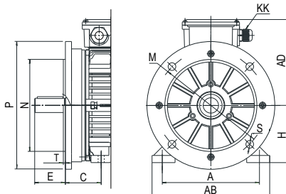
B35 (IM 2001)
