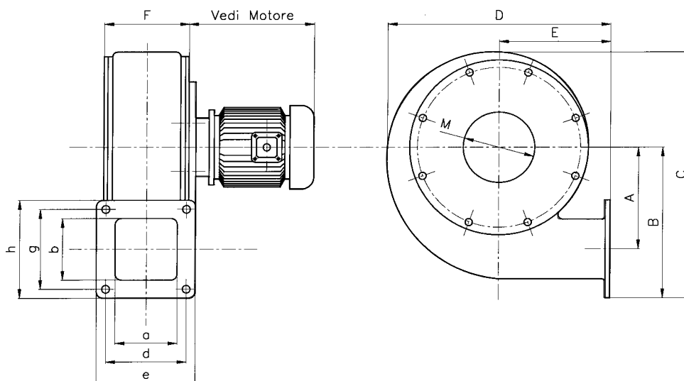
Dimensioni d'ingombro chiocciola (per dimensioni motore vedi pag. 300) Dimension of thread (for dimension of motors, see page 300) Platzbedarf spiralgehäuse (für motorabmessungen siehe seite 300) Encombrement carcasse (voir page 300 pour les dimensions moteur) Dimensiones exteriores de la carcasa (para las dimensiones del motor véase la página 300)
